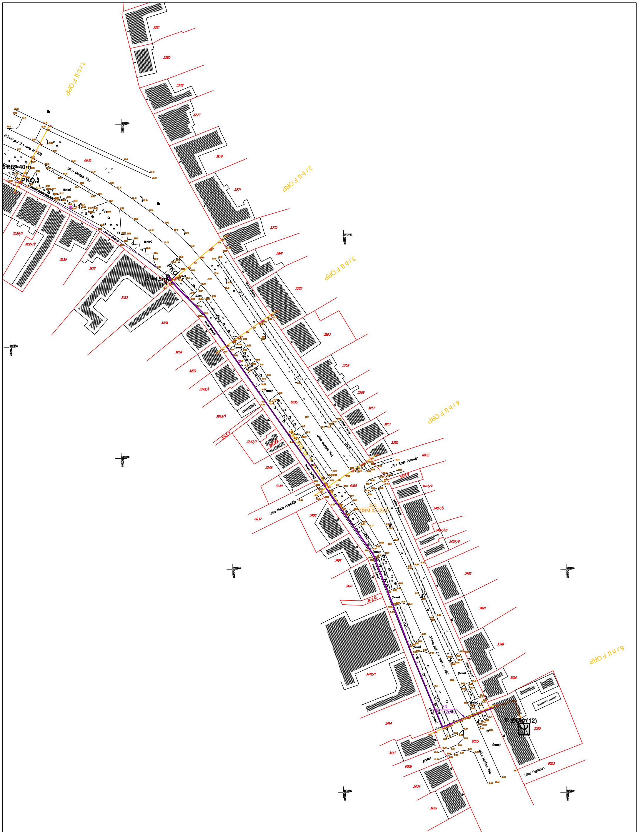
SITUACIONI PLAN R=1:1000
